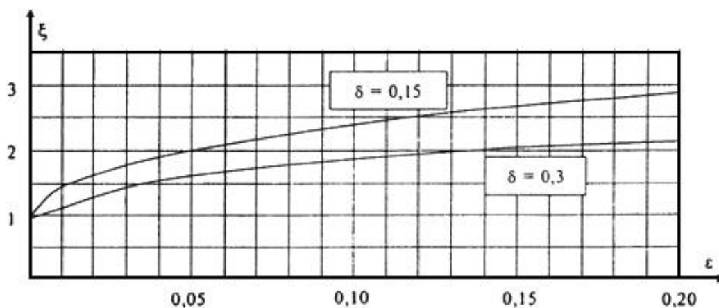
Рисунок 11.1 - Коэффициенты динамичности
