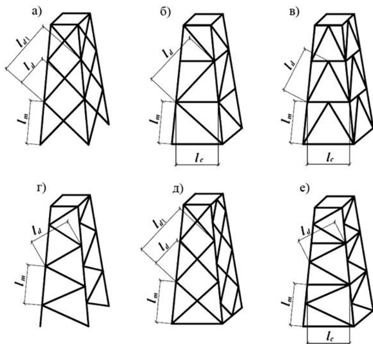
Рисунок 15 - Схемы пространственных решетчатых конструкций
