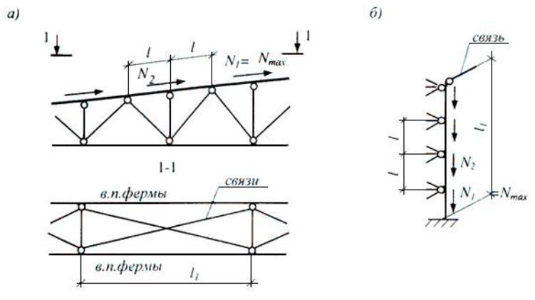
а - пояса фермы; б - ветви колонны
