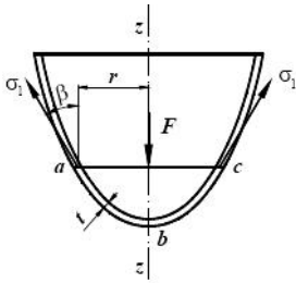
Рисунок 16 - Схема оболочки вращения
