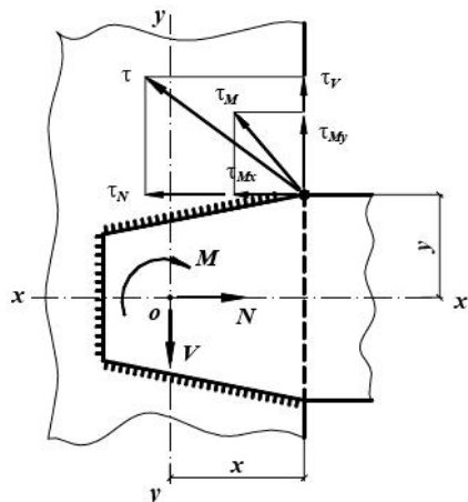
Рисунок 21 - Расчетная схема сварного соединения
