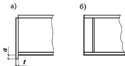
Рисунок 11 - Схема опорного ребра жесткости
