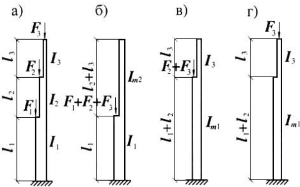
Рисунок И.1 - Схема двухступенчатой колонны (а) и условные схемы нагружений при приложении сил F_1, F_2 и F_3 соответственно к нижнему (б), среднему (в), верхнему (г) участкам
