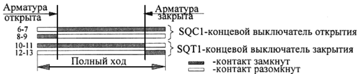
Рис.5. Электрическая схема соединения электромагнитов управления и концевых выключателей отсечной пневмоприводной быстродействующей арматуры (нормально закрытой и нормально открытой) при установке под оболочкой и вне оболочки
