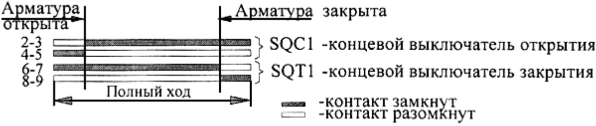
Рис.1. Электрическая схема соединения концевых выключателей арматуры с ручным управлением
