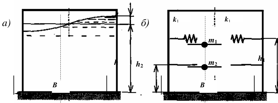
Рис.П.5.1. Моделирование резервуара с жидкостью:
