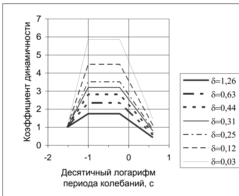
Рис. П.3.1. Спектры коэффициентов динамичности для различных логарифмических декрементов колебаний \delta
