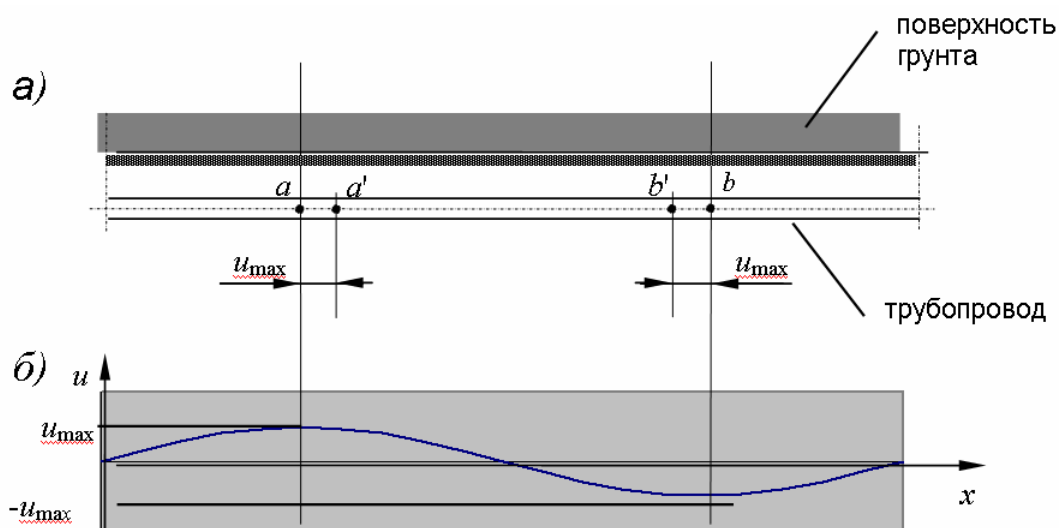
Рис.П.6.1. Деформации линейно-протяженной конструкции при прохождении продольной сейсмической волны:
