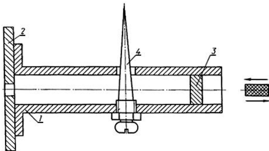
1 - волновод (10х23); 2 - диафрагма; 3 - поршень настройки; 4 - антенна
