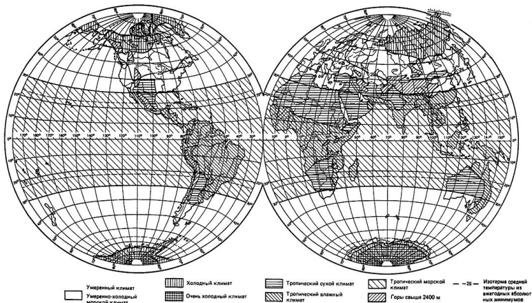
Макроклиматические районы земного шара
